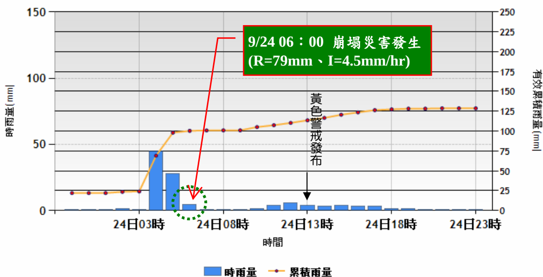
三和雨量站 降雨組體圖
